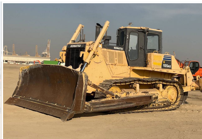
2013 KOMATSU D155AX-6
