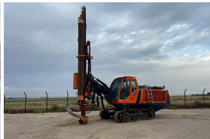
SANDVIK TITON 500
